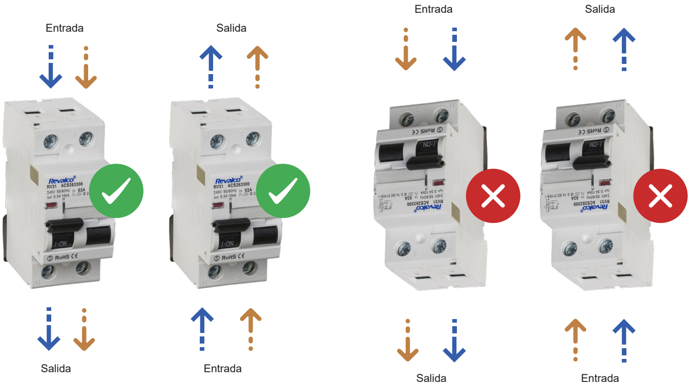
Instalación correcta
